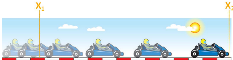
Doc.1 Chronophotographie du mouvement du kart.
